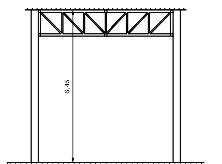
SEZIONE A-A
