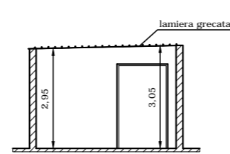
SEZIONE A-A
