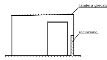
PROSPETTO D
